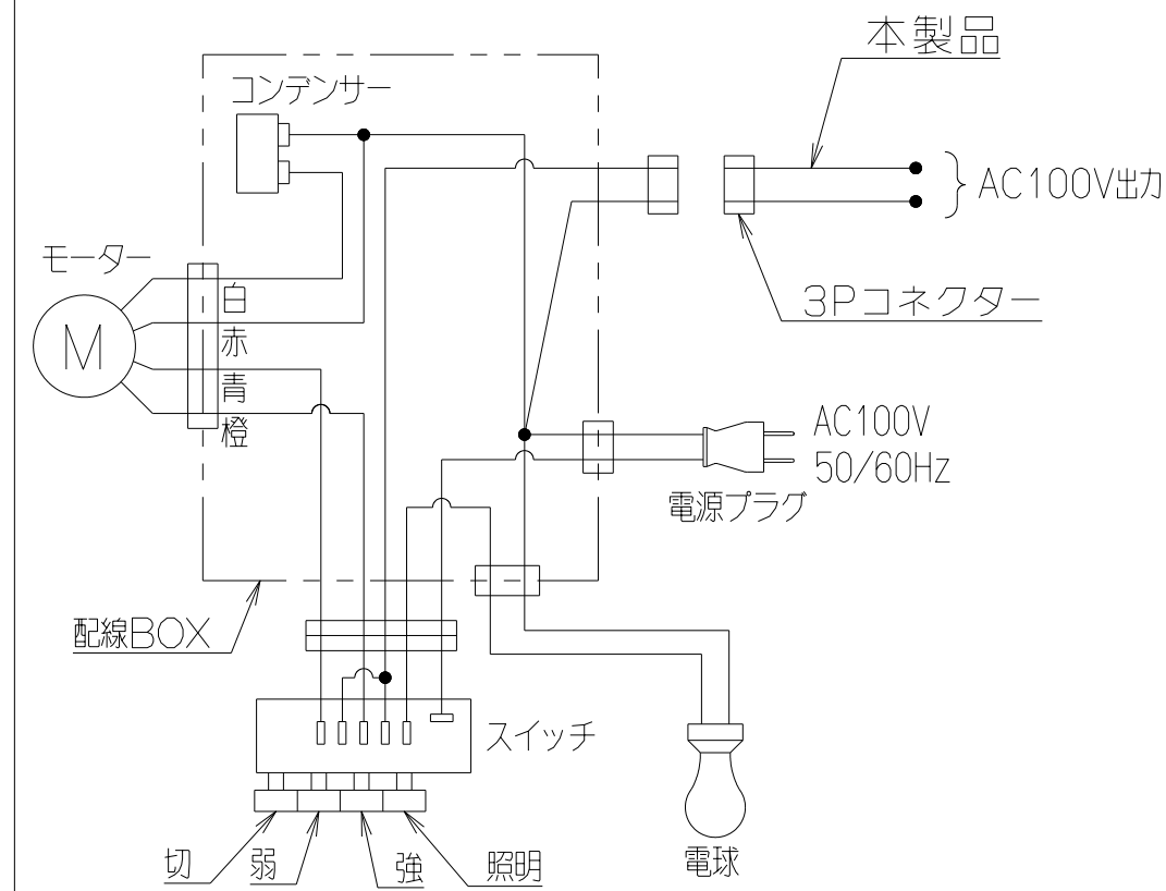
結線図 (レンジフード接続例)
